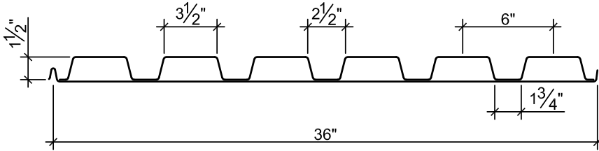
PLB-CD, PLB-CD AC, HSB-CD or HSB-CD AC
